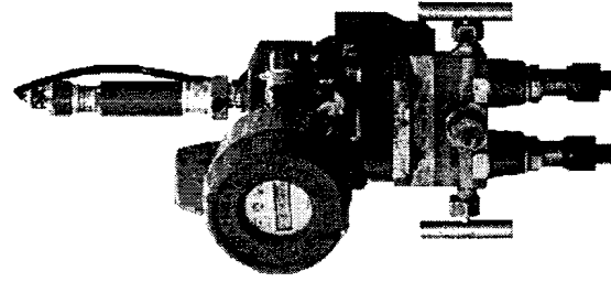
Рис. 27. Датчик «ГиперФлоу-3Пм» с вентильным блоком
