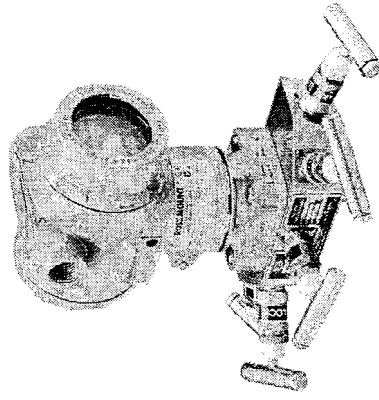
Рис. 29. Датчик 3095 MV с пятивентильным блоком
