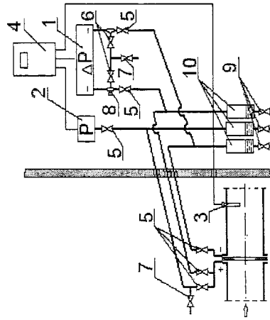
Рис. 16. Схема подключения средств измерений при измерении расхода газа:
