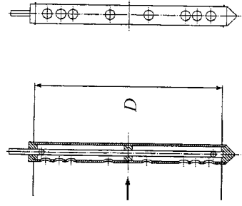
Рис. 22. Цилиндрическая усредняющая напорная трубка
