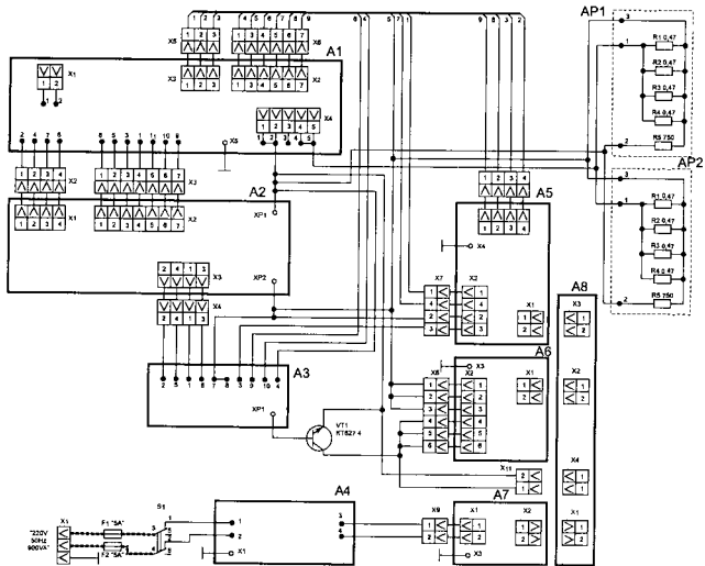
Электрическая схема межблочных соединений источника питания Б5-71
