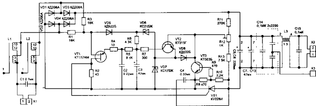
Принципиальная схема стабилизированного выпрямителя напряжения сети
