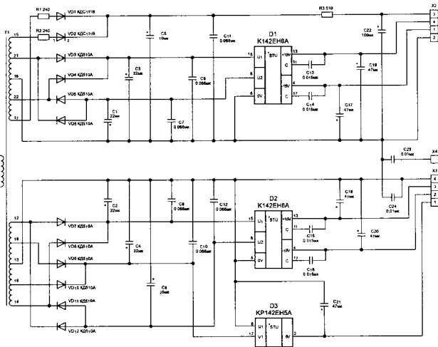
Принципиальная схема вспомогательных источников питания
