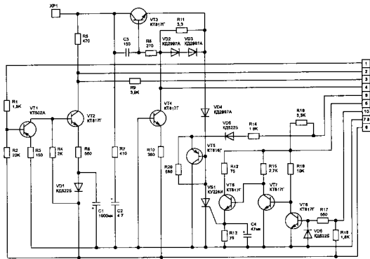
Принципиальная схема усилителя мощности и схемы регулируемой защиты выхода
