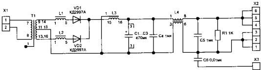
Принципиальная схема силового выпрямителя
