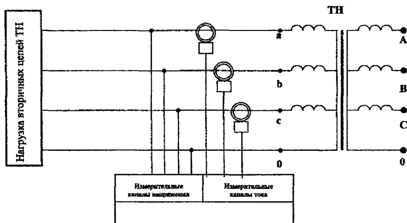
Рисунок 1 - Схема выполнения измерений мощности нагрузки трехфазного ТН
