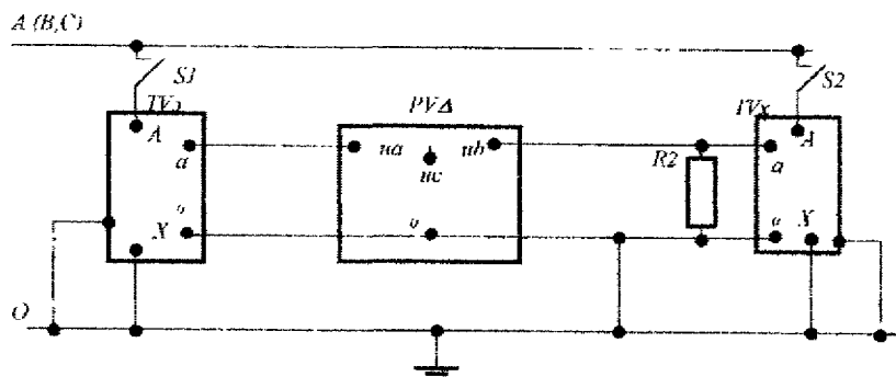
Рисунок 1 - Схема выполнения измерений мощности нагрузки трехфазного ТН
