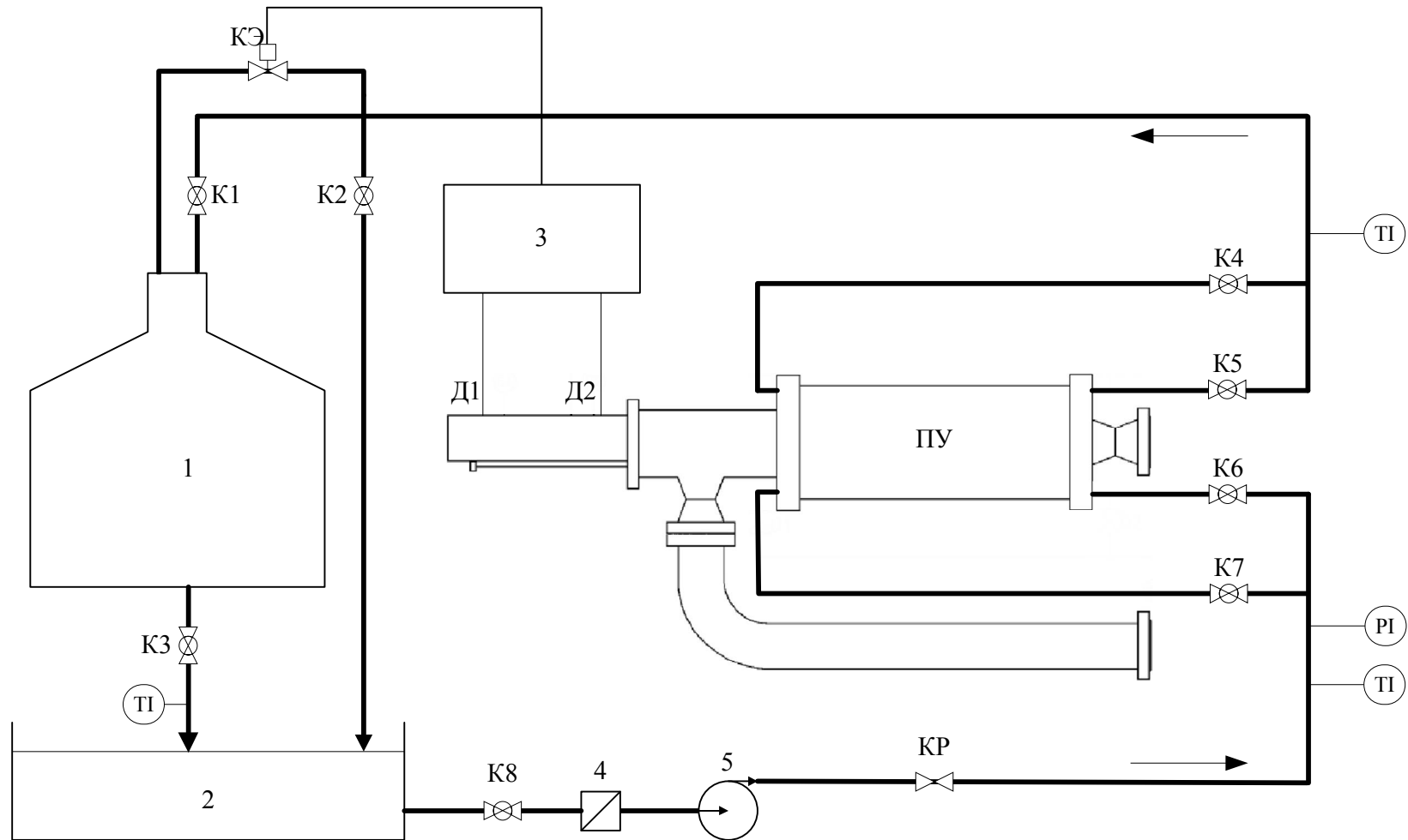
Рисунок А – Принципиальная схема соединений поверяемой ПУ и средств поверки
