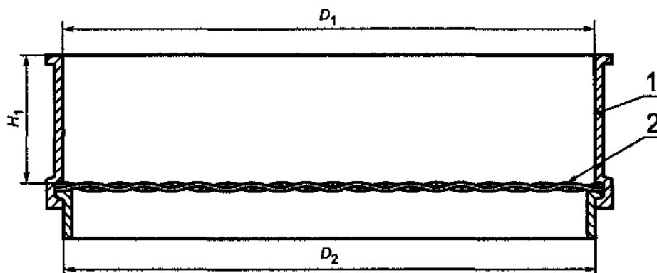
Рисунок 2 - Поперечное сечение лабораторного сита
