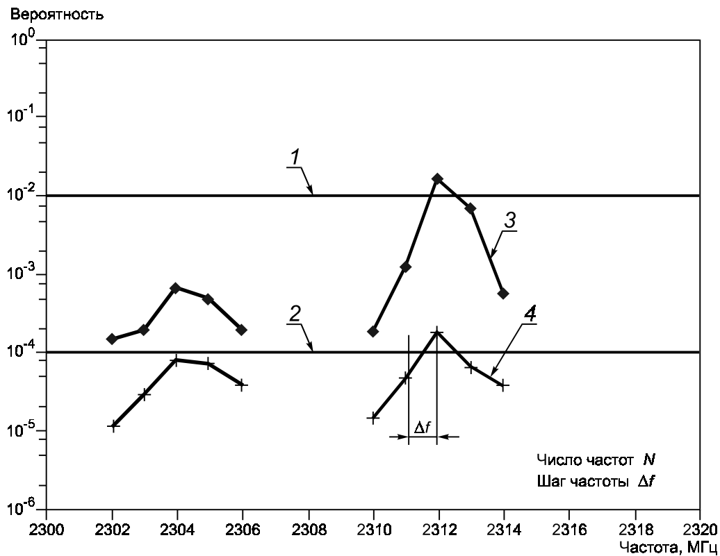
1 — P_{limit} при 60 дБ (1 мкВ/м); 2 — P_{limit} при 90 дБ (1 мкВ/м); 3 — P_{meas} при 60 дБ (1 мкВ/м); 4 — P_{meas} при 90 дБ (1 мкВ/м)
