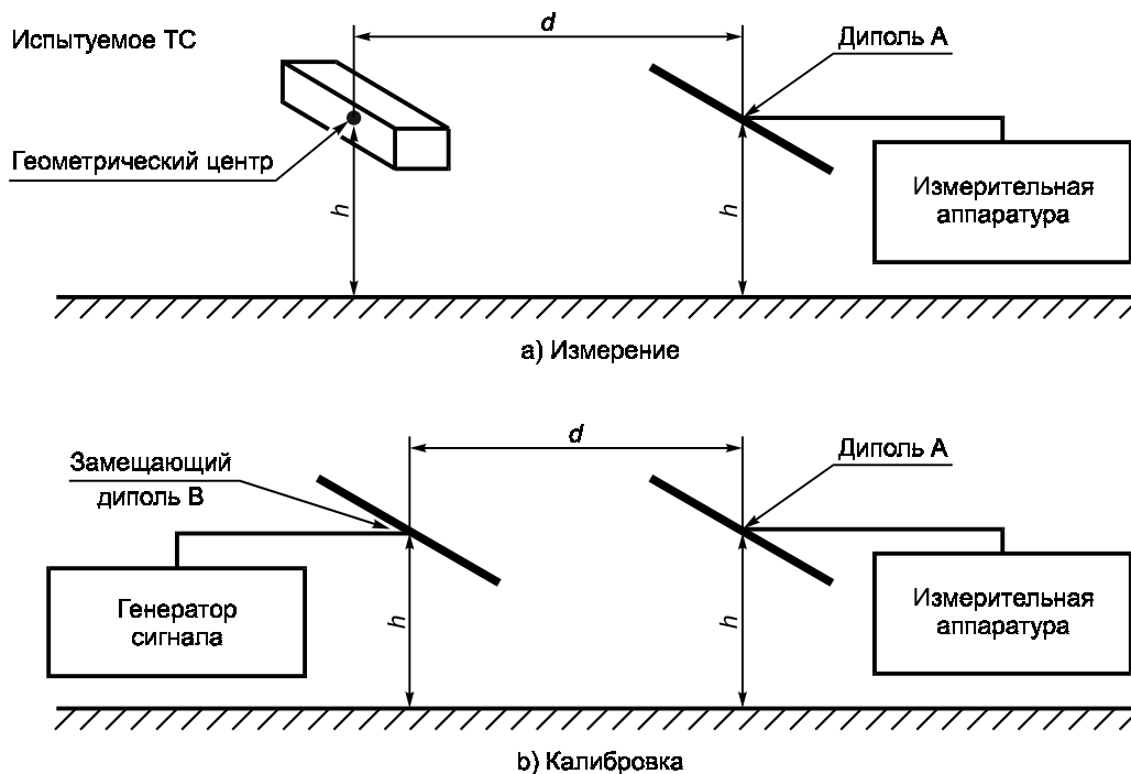
Рисунок 16 — Измерение методом замещения (см. 7.4.1 и 7.4.3)
