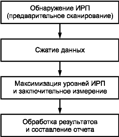
Рисунок 19 — Алгоритм проведения измерений
