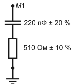
Рисунок 12 — Элемент RC для эквивалента руки (см. 7.4.2.3)
