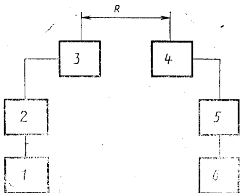
Состав и размещение ИА при контроле уровня излучаемого электромагнитного поля рамочными и дипольными или рупорными антеннами при отсутствии экрана
