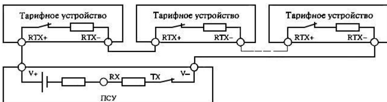
Рисунок 1б - Схема двухпроводной линии с несколькими исполнителями
