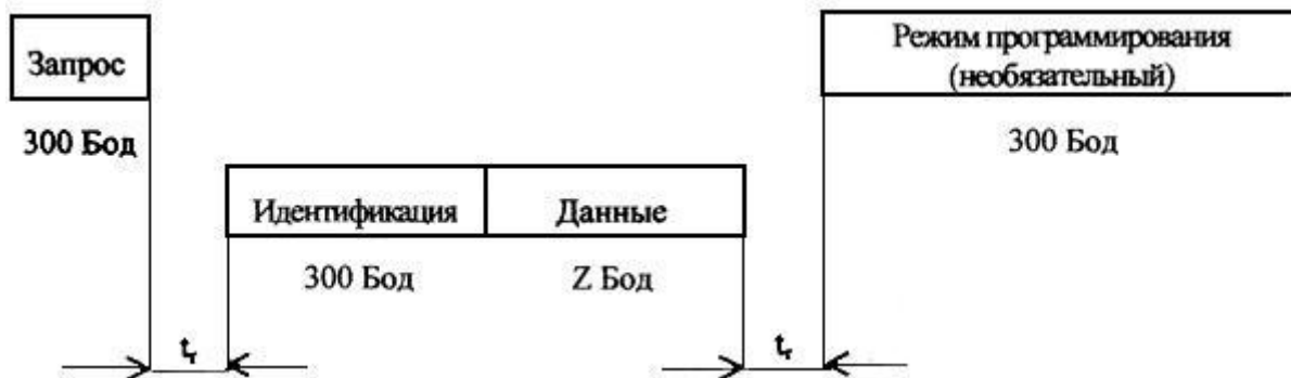
Протокол передачи для режима А
