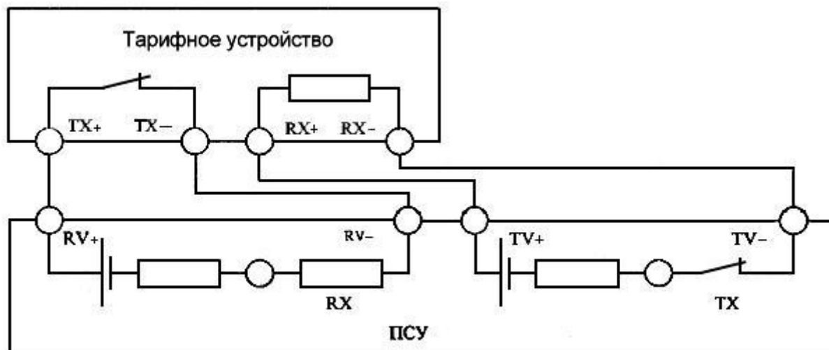
Рисунок 1с - Схема четырехпроводной линии с одним исполнителем
