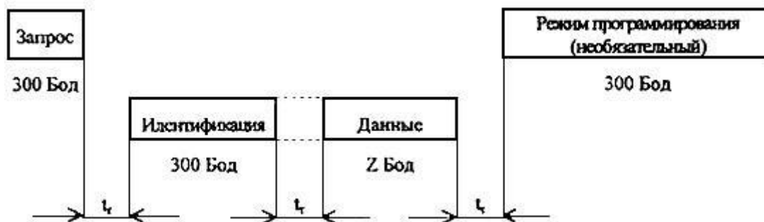
Протокол передачи для режима В
