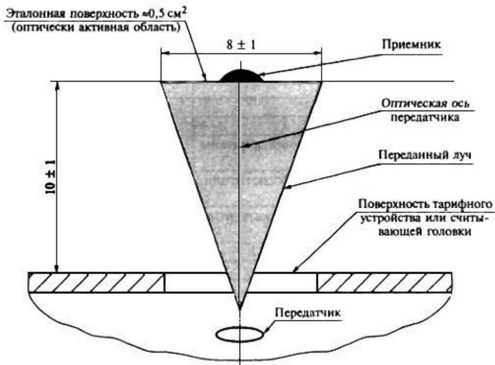
Рисунок 5 - Расположение передатчика при испытании
