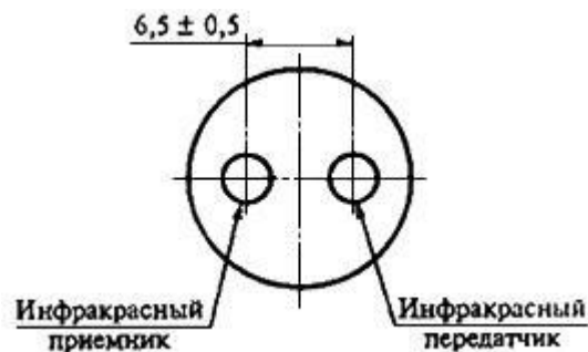
Рисунок 4 - Вид на оптический порт
