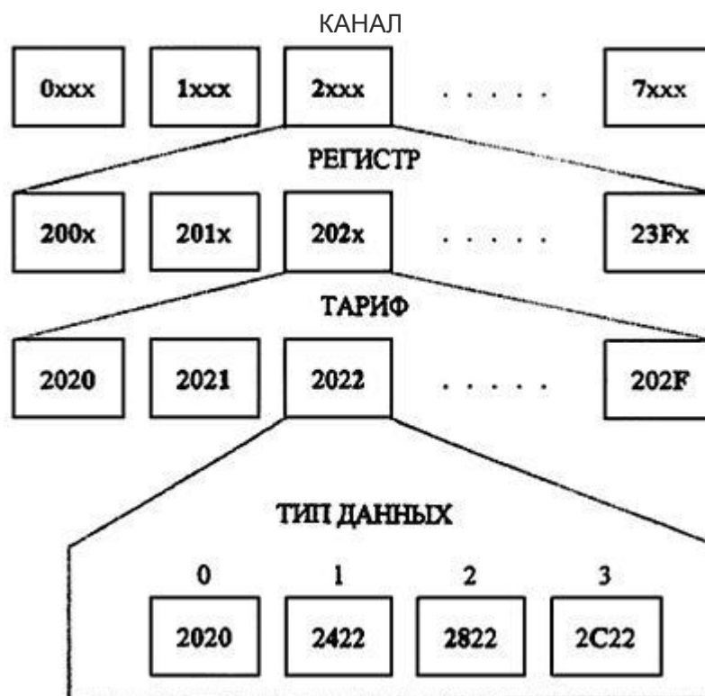
Рисунок С.2 - Диаграмма кодирования регистров
