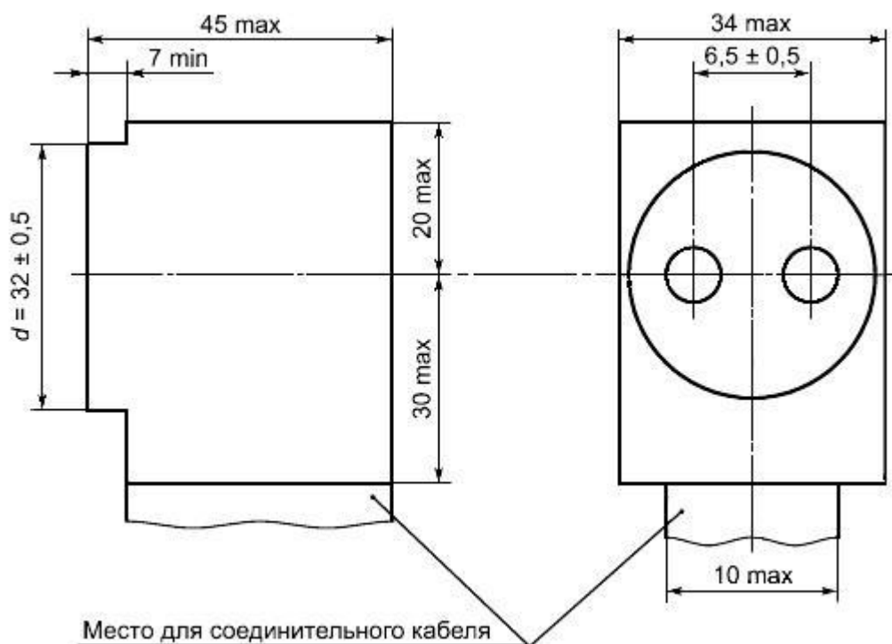
Рисунок 2b - Размеры считывающей головки
